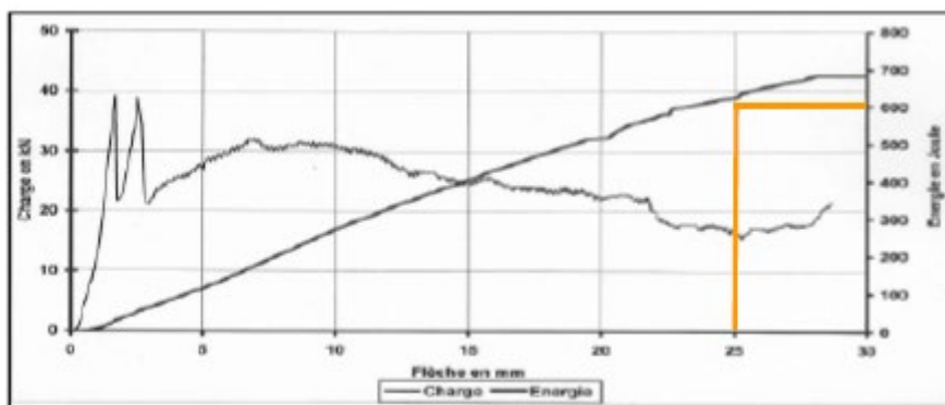
Curva di rottura/spostamento – Energia/spostamento CHRYSO®Fibre S50 a 4 kg/m 3 Prove Sigma Bétons
